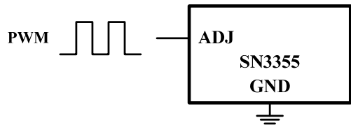
图17 ADJ引脚PWM信号调光
