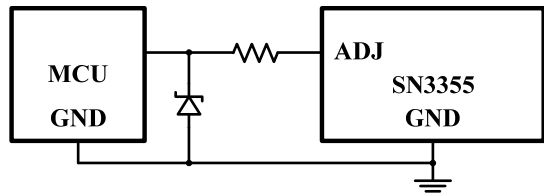
图18 ADJ引脚MCU调光
